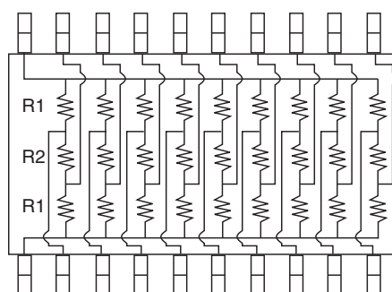
RDB: 20 pins
