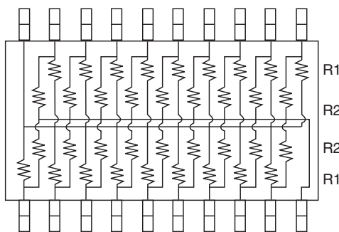
RDA: 20 pins
